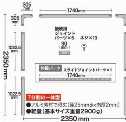
KIS23956 スライドゲート アーチフレーム ロット：1 セット
