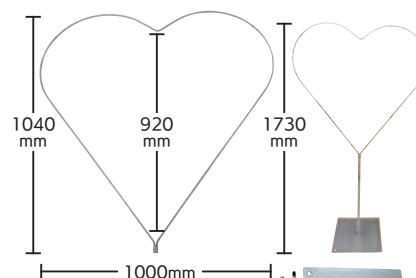
KIS22902 ハートフレームスタンド
