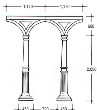
●スペイン柱 (2対) ¥36,000 内訳 柱 ¥12,000×2 05070 センターアーチ ¥6,000×2 05078
