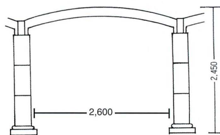
●オリエントアーチ (1対) W.3600 ¥32,000 内訳 柱 ¥12,000×2 05070 ジョイントアーチ ¥8,000 05078
