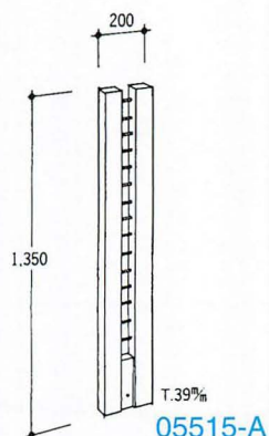
-AW 柱 (白染) H.1350 05515-A ¥3,300
