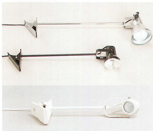
03711-1 (AM9564-A) 03711 W.600~700 レフ球 100W ¥2,500 03711-2 (AM9564-B) W.600~700 ハロゲン球 85W ¥3,800 03711-3 W.200~ 白 ハロゲン球 85W ¥2,500
