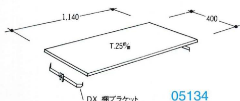
-A センター棚板 05134 CL クリヤー CW 白染色 ¥1,000
