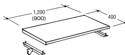
-ACL 棚板(栓クリア) (W1200) ¥1,000 05134 -BCL 棚板(栓クリア) (W900) ¥1,000 05134 -APW 棚(白合板) (W1200) ¥800 05134 -BPW 棚(白合板) (W900) ¥800 05134
