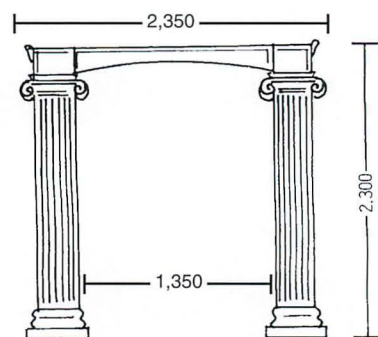
●ギリシャアーチ (1対) W.2350 ¥46,000 内訳 柱 ¥15,000×2 05070 ジョイントアーチ ¥8,000 05078 ジョイントボックス ¥4,000×2 05079
