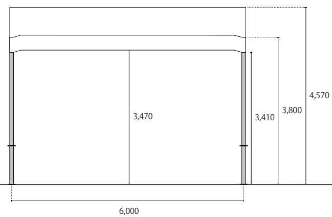
【側面】
