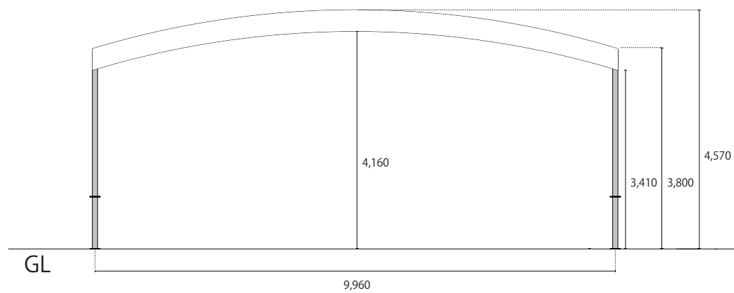
【正面】
