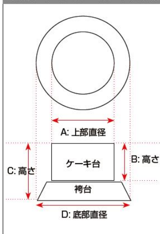
袴台付ウェディングケーキ台 サイズ詳細
