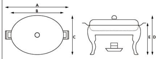
小判チェーフィング シングル サイズ詳細
