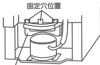
蒸発皿
