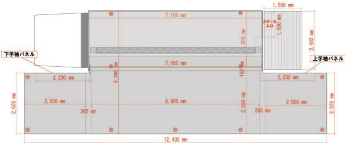
BH盛岡ライブステージカー <ステージ寸法図面(展開時)>
